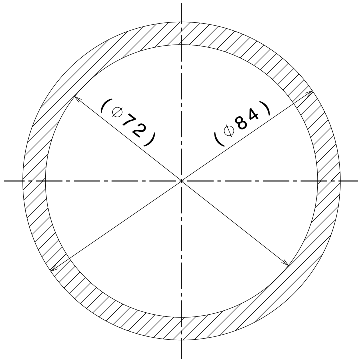
SEALING FACE TEMPLATE 'RING' Scale: 1:1
